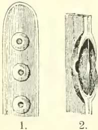
1. Gehöfte Tüpfel. 2. Ein Tüpfel im Durchschnitte, noch stärker vergrößert (schematisch).
