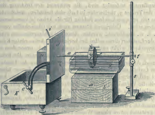
Fig. 33. i ist der zum Aufziehen der Uhr dienende Hebel; h sind untergestellte Holzklötze. — Um ein rückweises Drehen zu vermeiden, das jede Pendel- und Ankeruhr hervorbringt, dient mir ein durch Flügel regulirter, übrigens ähnlich gebauter Apparat, der Drehungen sehr verschiedener Schnelligkeit herzustellen gestattet.
