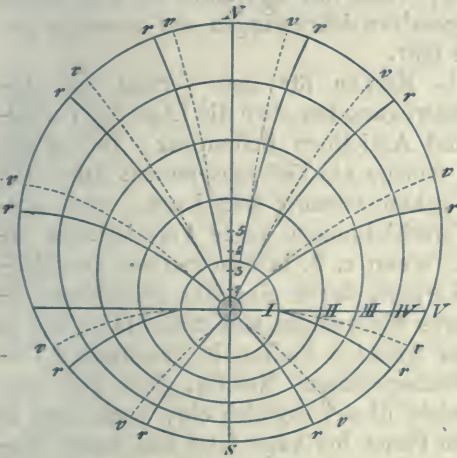
Fig. 11. Als Grundlage der Construction diente ein System nicht concentrischer Kreise, deren Mittelpuncte auf der Symmetrieachse NS bei 2, 3, 4, 5 liegen. (Nach Sachs.)
