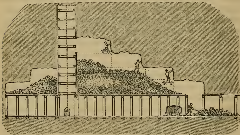
Fig. 1. BEWERKING MET OMGEKEERDE TRAPPEN.
