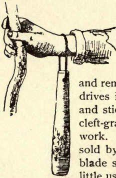
130. Grafting-mallet (XI-10).
