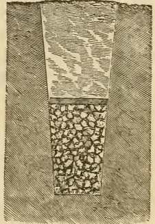
Fig. 1.—RUBBLE DRAIN.
