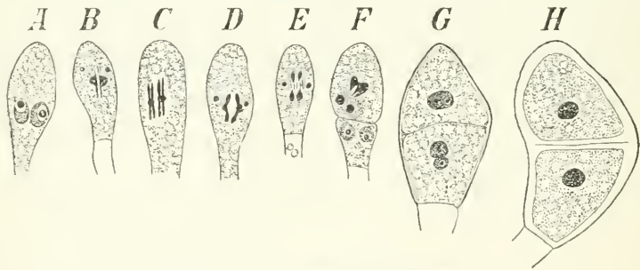
Fig. 22. Puccinia liliacearum .
