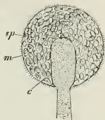
Fig. 42. Mucor mucedo .
