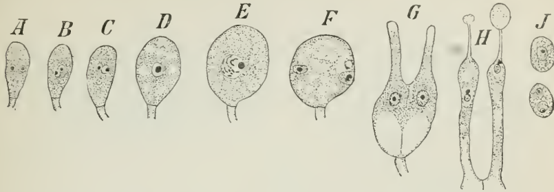
Fig. 23. Tremella mesenterica .
