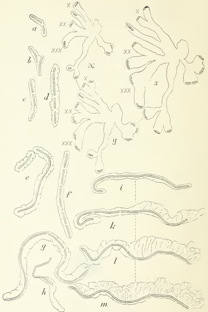
Fig. 7. Bacterium vermiforme .
