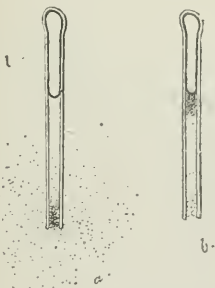
Fig. 67. Chemotaxis.
