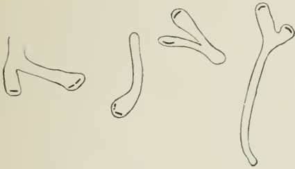
Fig. 6. Bacterium pediculatum.
