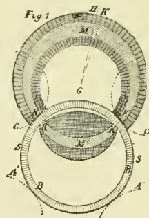
FIG. 1.—Sir W. Thomson's Roller Dynamo.
