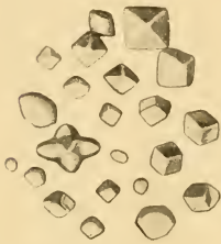
Fig. 21. Kristalle von Ammonium- phosphomolybdat. Vergr. 350.
