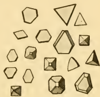
Fig. 28. Kristalle von Silberchlorid. Vergr. 400.
