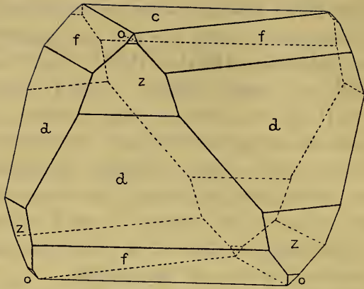
Fig. 7. Steenstrupite, type III.
