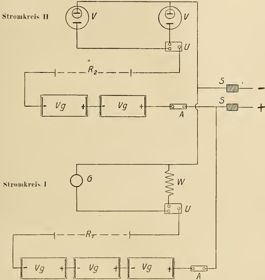
Schaltungsskizze.
