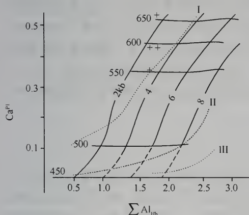
图6 斜长石-角闪石实验地质温压计 (Plyusnina 1982) I: 低压相系; II: 中压相系; III: 高压相系
