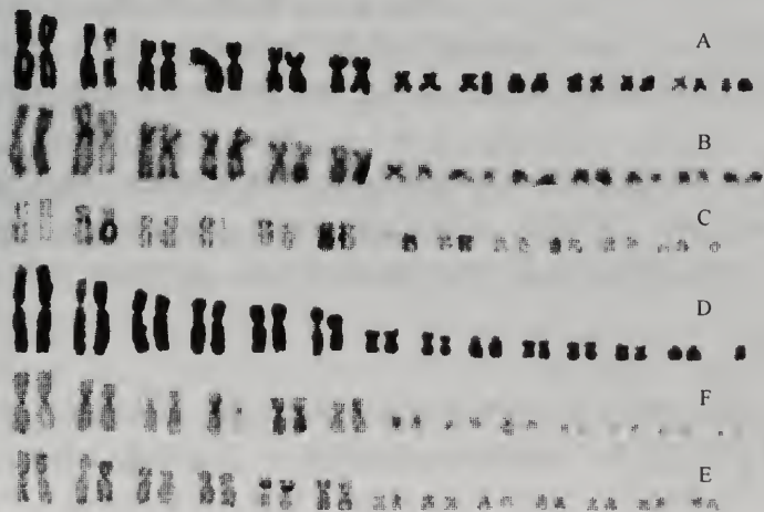
图 1 高黎贡山白颌大角羚的核型、C 带及 Ag-NOR
