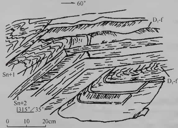
图 4 瑞丽勐典 D_1 -f 斜歪水平褶皱及斜卧褶皱共生（据南京里剖面 51 层）
