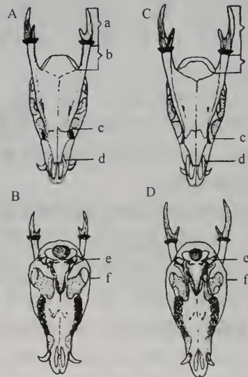
图 1 新种与菲氏鹿的头骨比较
