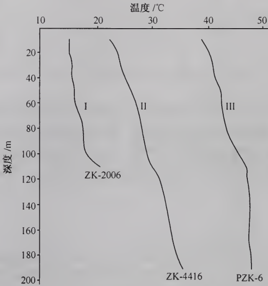
图 2 三种温度-深度曲线类型
