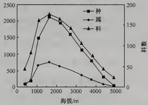
图 3 科属种丰富度随海拔梯度的变化
