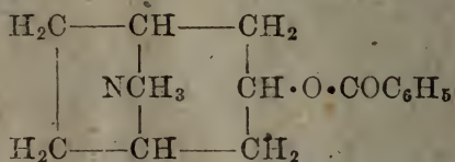
託 派 古 柯 碱
