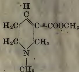
檳榔硷
