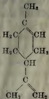
右-檸檬萜
