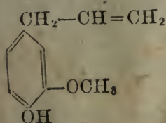
丁香油酚
