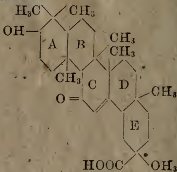
甘草次酸 (Ruzicka)
