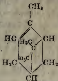
左-松节油萜
