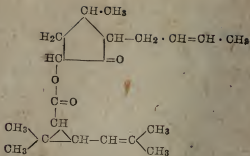
除虫菊素 I
