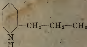
2-丙基胡椒啶
