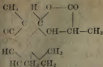
山道年 (Ruzicka, 1930)
