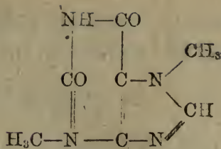
柯柯豆硷
