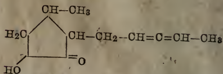
除虫菊酮
