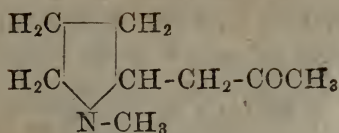
α-海 癡 林
