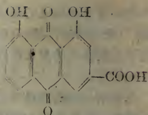
氧化大黄酸
