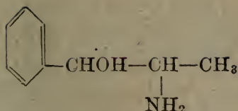
左旋-去甲基麻黄硷
