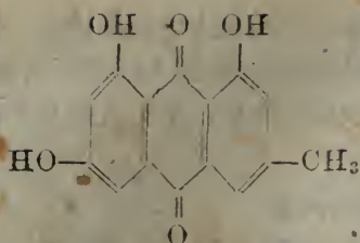
大黄泻素
