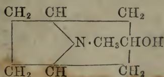
託品
