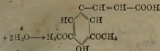
白芥子硷酸
