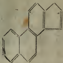
环戊烯-菲
