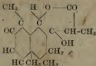
苦艾素 (Tettweiler, 1932)
