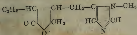
毛果芸香硷
