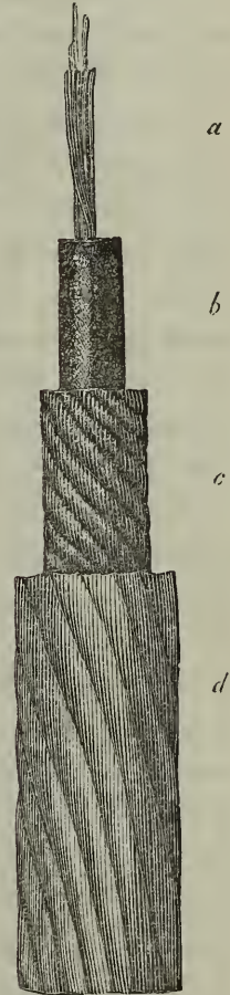
Fig. 7. Stuk van den Transatlantischen kabel; nat. gr.; a. 7 koperdraden, tezamen gedraaid en dienende tot geleider; b. gutta-percha bekleeding; c. bedekking van geteerd touw; d. 18 ijzeren touwen, ieder 7 draads, vormende de buitenste laag.
