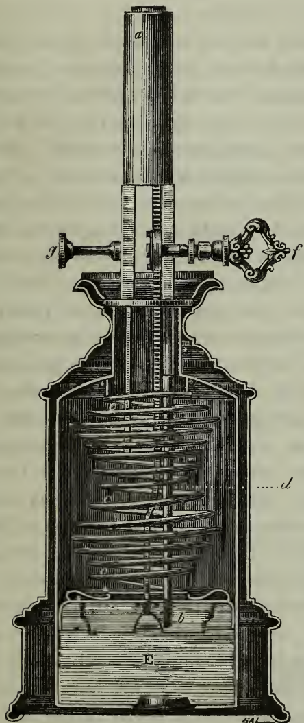
Fig. 6. Moderateurlamp in doorsnede. a buis voor het kousje. b zuiger, die de olie naar beneden perst door de drukking van ccc eene spiraalveer. d buis, waardoor de olie in de ouis a wordt opgeperst. E reservoir. f sleutel om de veer ccc op te winden. g rondsel om het kousje hooger of lager te stellen.
