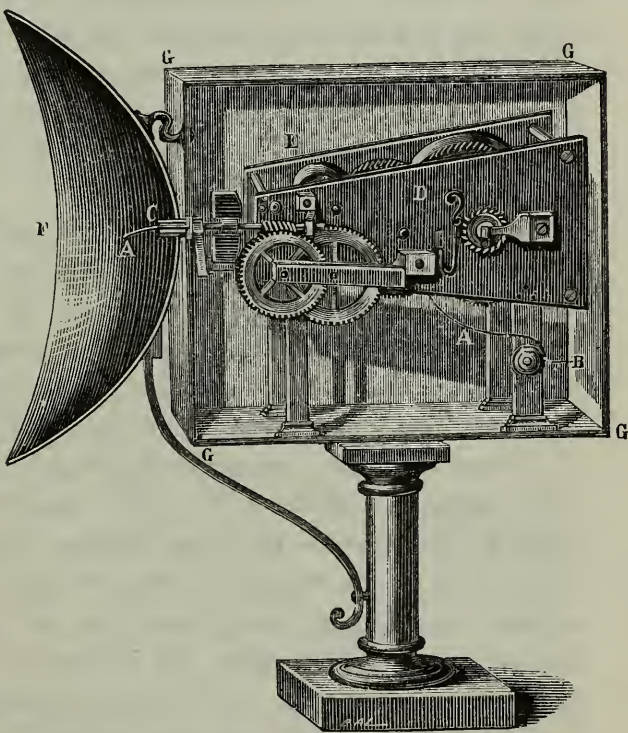
Fig. 15. Magnesiumlamp met uurwerk.
