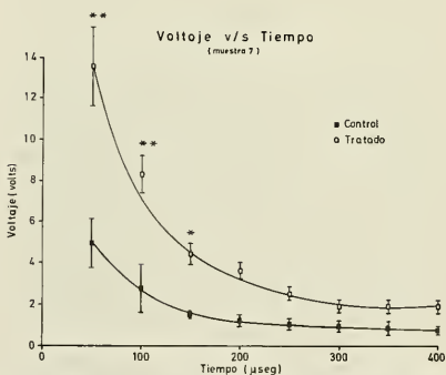
FIGURA 4. Curvas voltaje-tiempo obtenidas aplicando pulsos eléctricos cuadráticos para generar la respuesta cortical directa (RCD).
