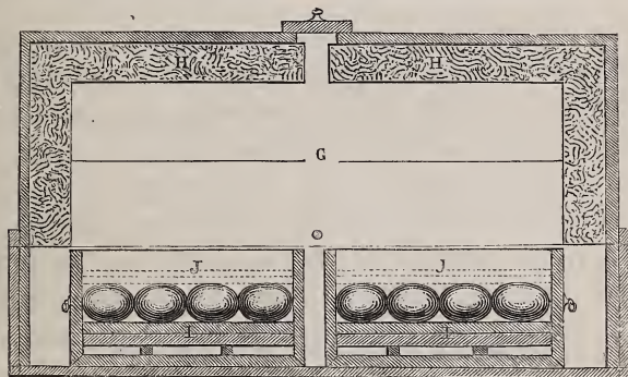
Coupe intérieure du couveroir.
