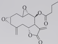
cordifine
