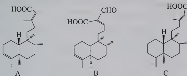
常山烷二萜
