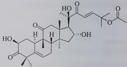
cucurbitacin B
