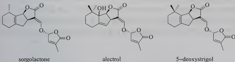
sorgolactone
