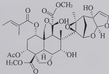
azadirachtin
