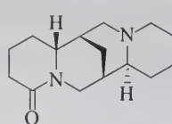
lupanine
