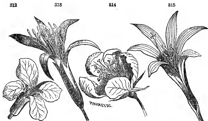
Forms of corollas. 312, Cheiranthus (stock). 313, Silene regia (scarlet catchfly). 314, Pyrus coronaria . 315, Amaryllis (Atamasco lily).
