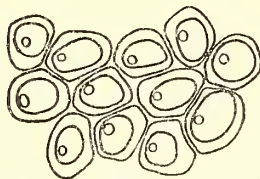
FIG. 39. Saissetia oleæ (Bern.), adult female, derm areolation, \times 165 .
