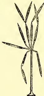
Dendryphium fumosum. Magn. 200 diams.
