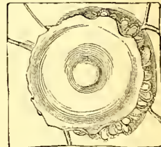
Aspidium trifoliatum. An indusium covering a sorus.
