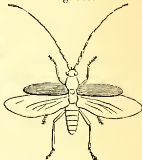
Cerambyx ædilis. Nat. size.
