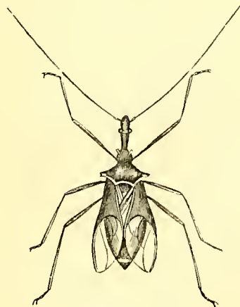
Reduvius tuberculatus. Nat. size.
