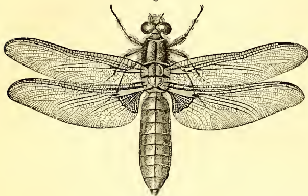
Libellula depressa. Nat. size.
