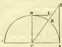
Cotangent.
