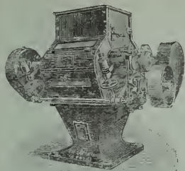
Moulin à cylindre "Diagonal"
