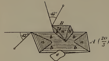
Fig. 4. Cristal de pyroxène longueur 4 millim.; de la leucite N° 6.
