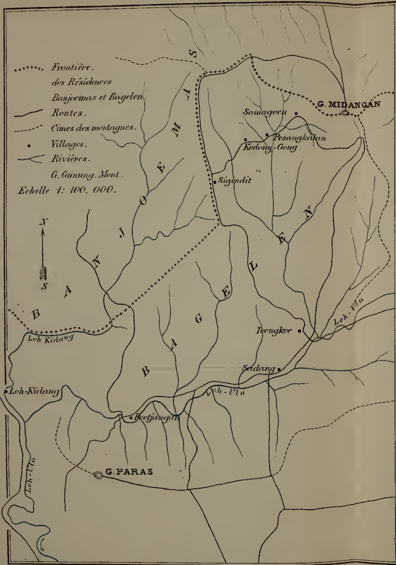
Fig. 1. Le terrain où se trouvent les schistes anciens près du mont Midangan, à la frontière de Bagelen et de Banjomas. Copie de la Carte topographique 1: 100.000.
