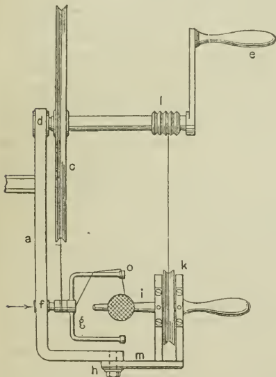
Steins Knäuelwickelmaschine.
