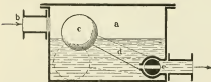
Kondensationswasserableiter.
