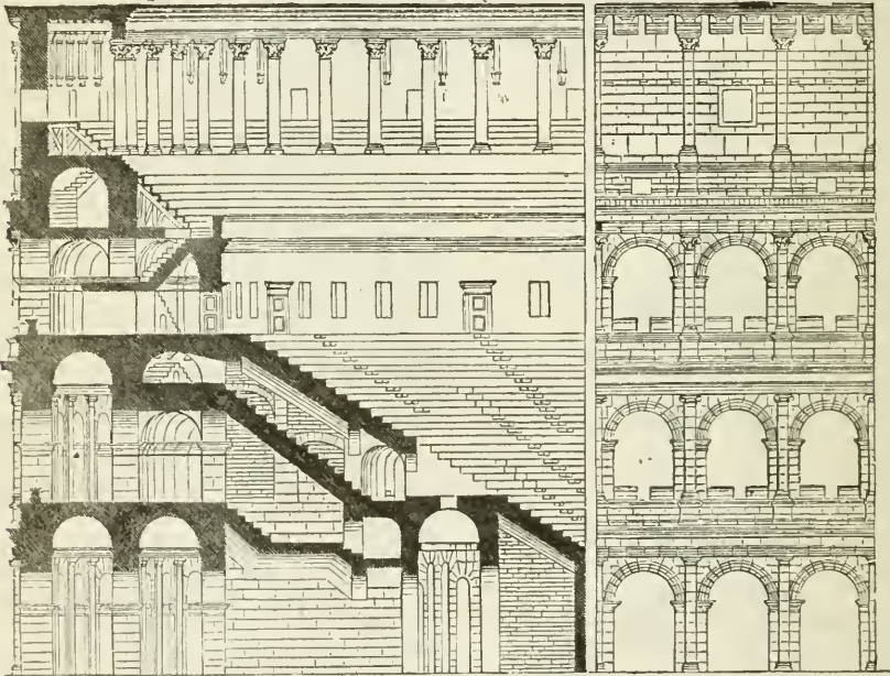
Durchschnitt und Teil vom Aufriß des Koloßeums in Rom.
