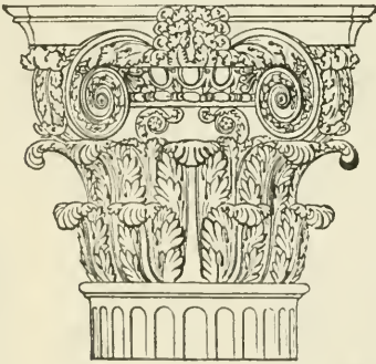
Kompositenkapitäl (vom Titusbogen in Rom).
