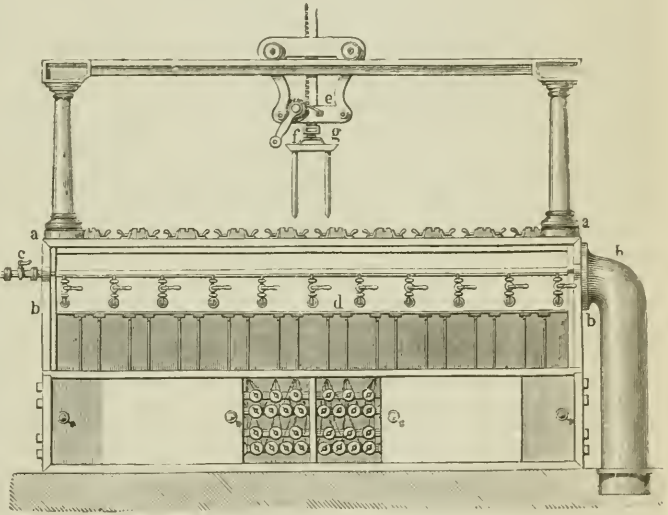
Gießmaschine für Stearinkerzen.
