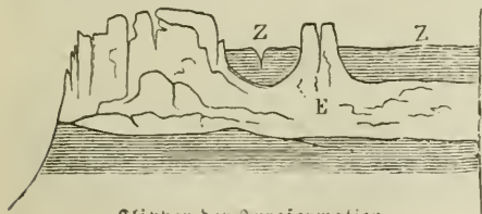
Klippen der Juraformation.
