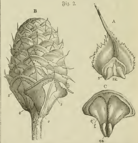
Edelkanne. A Deckblatt, B Stüd des reifen Zapfens, C reife, samentragende Schuppe, c Deckblatt, s Schuppe, sk Samentknospe, sa Same, f Anhang desselben.
