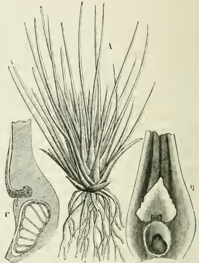
Brachsenkraut ( Isoetes macrospora ). A Ganze Pflanze (½ natürliche Größe) B Blattgrund mit dem Sporangium am Grund und darüber befindlichem Blättchlein. C Längsschnitt des Blattgrundes mit dem gesammerten Sporangium.
