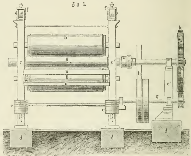
Dreiwelkliger Kalandar.
