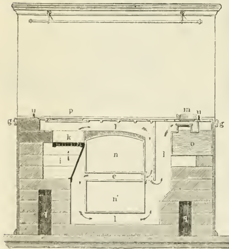
Wandkochmaschine.
