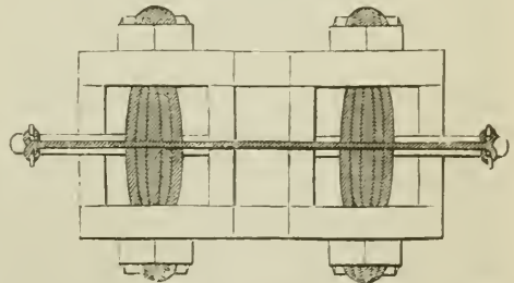
Spannrollen der Wurfgeschütze.
