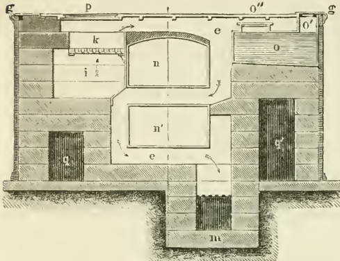
Kochmaschine von Adler, Durchschnitt.
