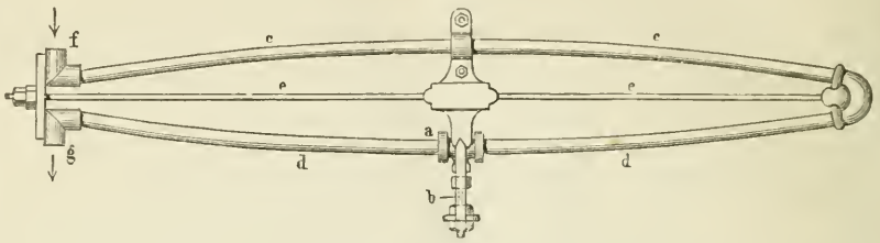
Rufenbergs Kondensationswasserableiter.
