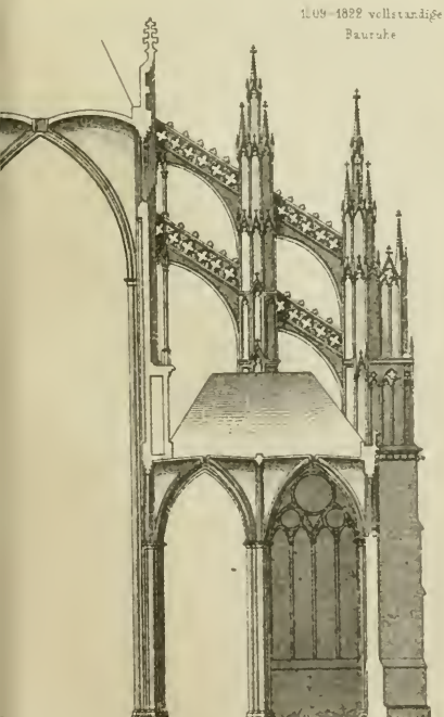
4 Ansicht der Strebepfeiler u. Strebepfeile
