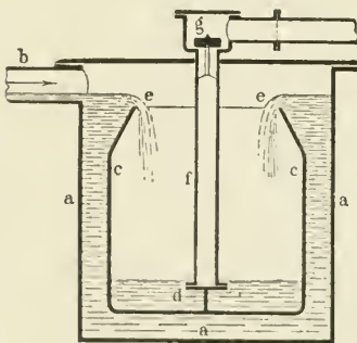
Kondensationswasserableiter.
