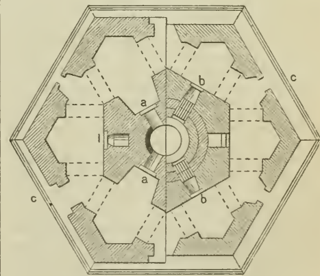
Rüdersdorfer Kalkofen (Grundriß).
