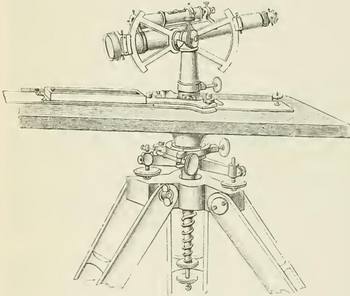
Meßtisch nebst Kippregel von Breithaupt in Kassel.
