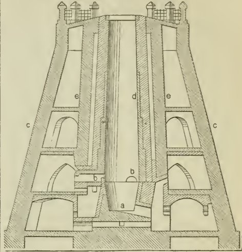
Rüdersdorfer Kalkofen (Durchschnitt).
