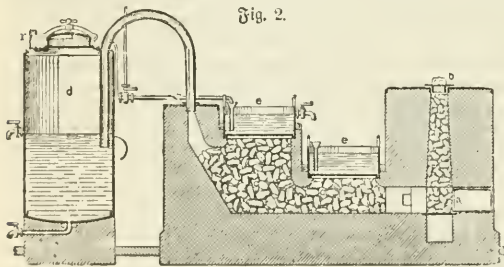
Rindler'scher Ofen.
