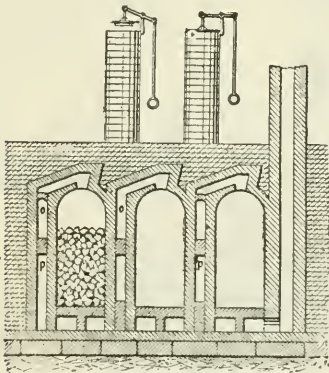
Smetscher Ofen.
