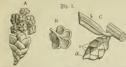
Eibe. A männliche Blüte, B Staubgefäß, C weibliche Blüte. b Nabel, s Knospenschuppe, sk Samentknospe.
