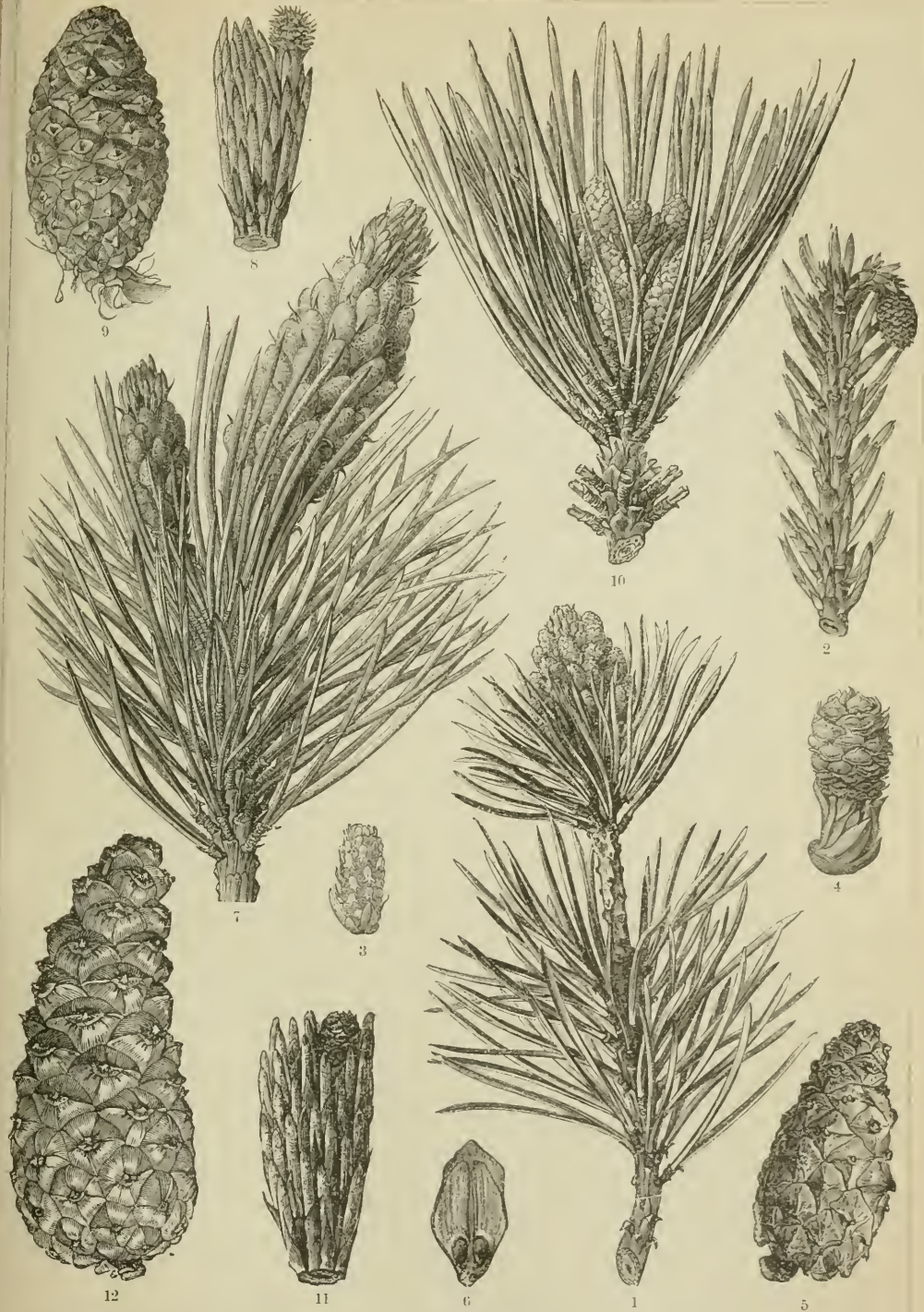
1—6 Gemeine Kiefer ( Pinus silvestris ). 7—9 Knieholzkiefer ( Pinus montana ). 10—12 Corsische Kiefer ( P. maritima ). 1, 7, 10 Triebspitze mit männlichen Blütenkätzchen; 2, 8, 11 mit weiblichen Blütenzäpfchen. 3 männlicher, 4 weiblicher Blütenstand. 5, 9, 12 Zapfen. 6 Samenschuppe mit zwei Samen.
