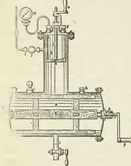
Kohlensäureentwicklungsapparat.
