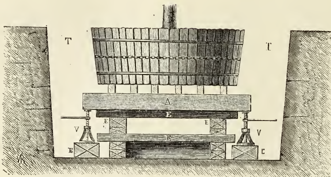
Fig. 50. — Système employé par M. Demouilles pour l'extraction du Cèdre.
