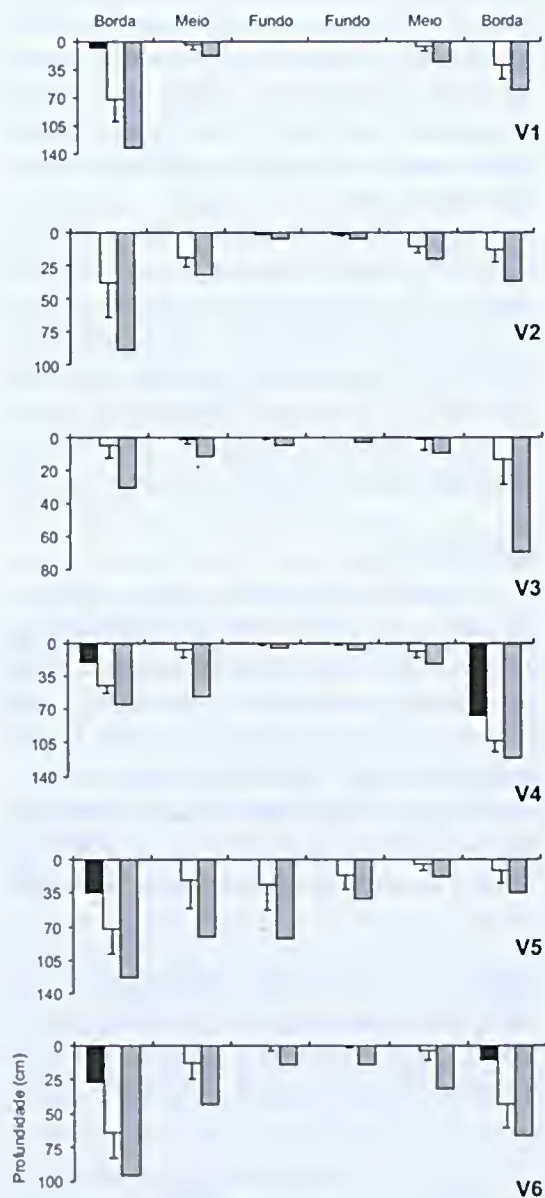
Figura 2 - Profundidade mínima ■, média □ e desvio padrão e máxima ■ do lençol freático nas três zonas (borda, meio e fundo) das veredas V1 a V5 em Uberlândia, e V6 em Uberaba, Minas Gerais, Brasil. n = 36.
