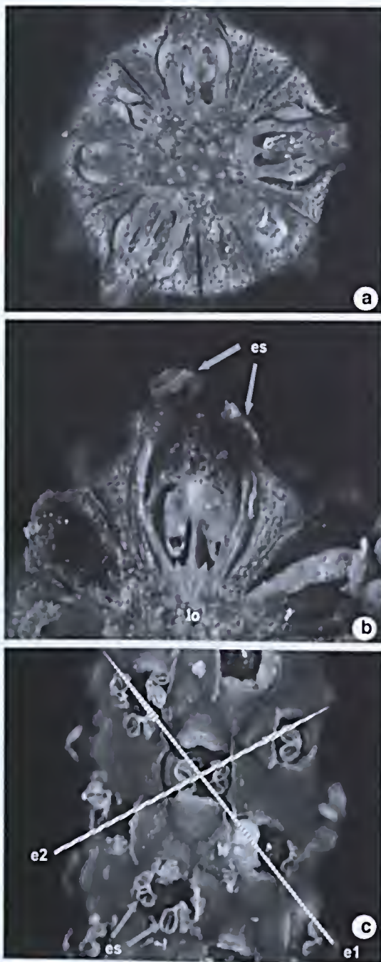
Figura 9 – a-c. Anthurium mareense – a. detalhe do espádice, em seção transversal; b. detalhe da flor, evidenciando estames excertos (es) e lóculos do ovário (lo); c. detalhe do espádice com os estames (es) excertos, mostrando o arranjo espiralado das flores em espiral principal (e1) e secundária (e2) ( Nadruz 1548 cultivado no JBRJ).
