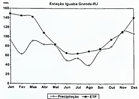
Figura 2 – Balanço hídrico com base em dados de 1970-1999, da Estação Meteorológica de Iguaba Grande (22°50'S, 42°10'W, 6 m alt.), localizada no centro do CDVCF, evidenciando o elevado déficit hídrico (324 mm), com a evapotranspiração potencial (ETP) (média anual de 1244 mm) superando a precipitação (média anual de 920 mm) em quase todos os meses do ano (Fonte: Freitas et al. 2005).
