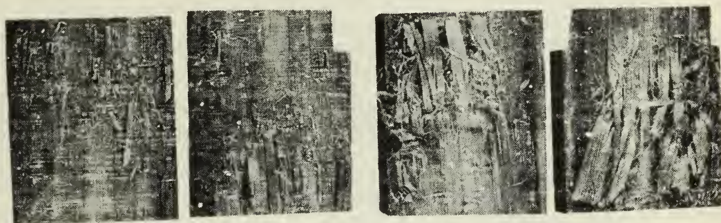
Fig. 12.— Failures in shearing parallel to grain tests for green motillo. (Fallas en los ensayos sobre deslizamiento paralelo al grano en el caso de motillo en estado verde).
