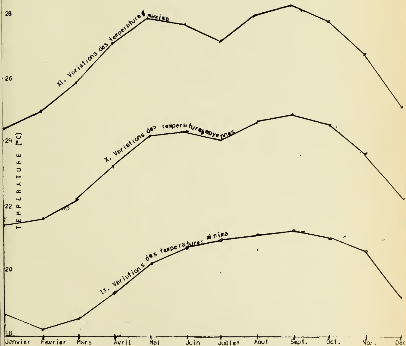
Fig. 15- Courbes des variations de temperature minima, moyenne et maxima, en secteur de forêt hygrophytique. (Curves of variations in minimum, average and maximum temperature in hygrophytic forests.) (Curvas de las variaciones en las temperaturas mínima, media y máxima, en sector de bosque higrofítico.)
