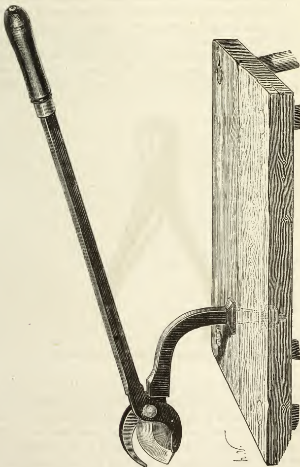
Fig. 114. — Étrancheur fixe.
