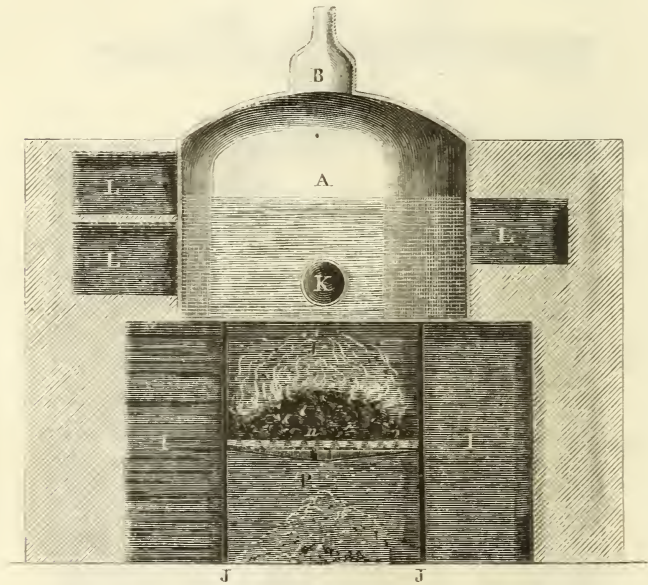
Fig. 56. — Appareil de chauffage à vapeur (coupe transversale).
