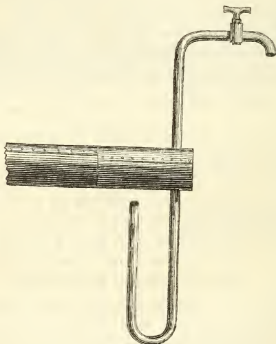
Fig. 67. — Échappement de la vapeur.
