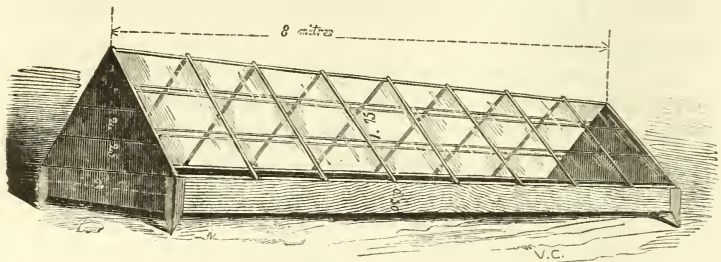
Fig. 66. — Châssis mobile.
