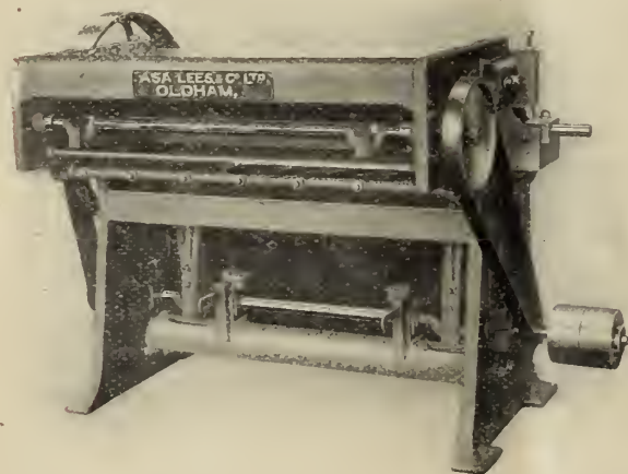
Fig. 22. — Egreneuse de coton à rouleaux, type Mac Carthy.
