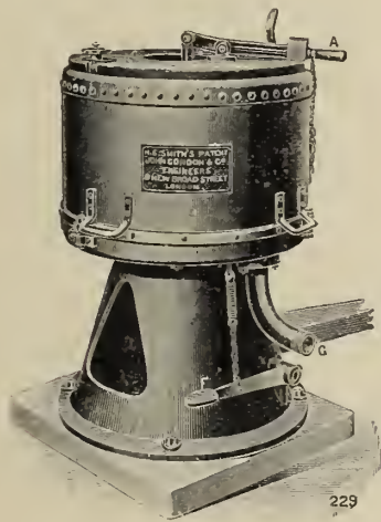
FIG. 45. — Séparateur centrifuge à latex.
