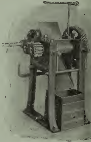
Laminoir laveur pour caoutchouc brut commandé à la main et par courroie.
