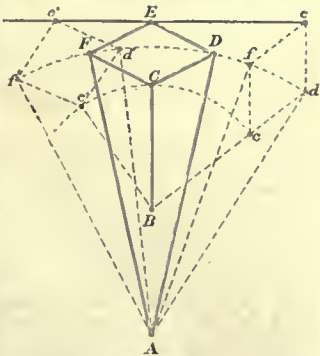
Peaucellier Cell.
