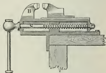
Fig. 13. Parallelschraubstock (Schnitt).
