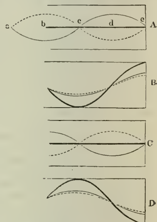
Fig. 4. Stehende Wellen in einer Röhre.
