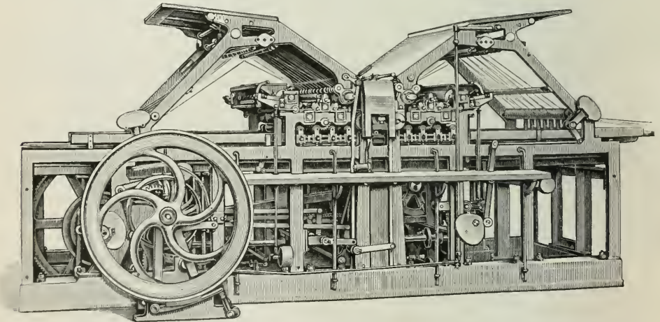
Fig. 7. Johannisberger Doppelmaschine für Illustrationsdruck mit schwingendem Druckcylinder und zwei Farbwerken.
