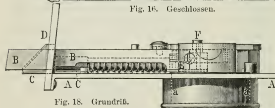
Fig. 16—21. Protectorschloß von Kromer.
