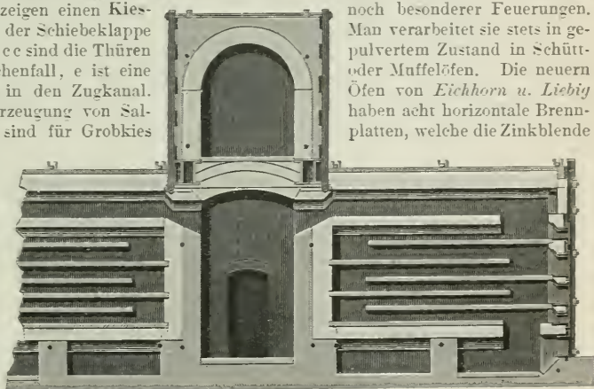
Fig. 3. Längsschnitt.
