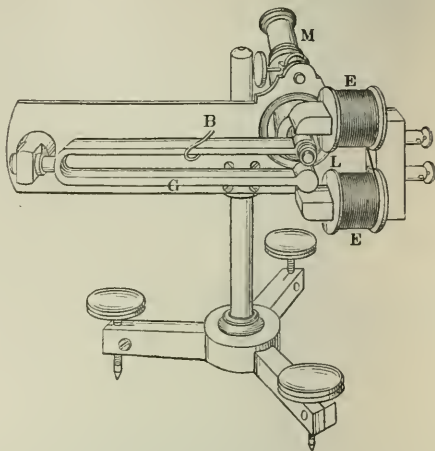
Fig. 20. Vibrationsmikroskop.
