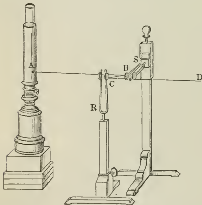
Fig. 19. Lissajous' optische Methode der Vergleichung von Stimmgabeln.
