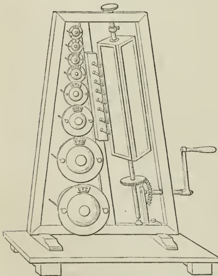
Fig. 26. Resonatoren-Flammenapparat.
