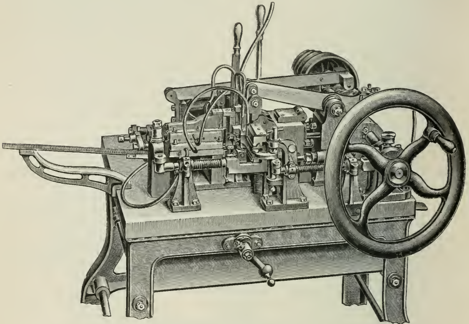
Fig. 2. Komplettgießmaschine von Küstermann u. Komp. in Berlin.
