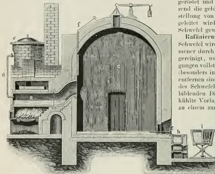
Fig. 4. Längsschnitt.
