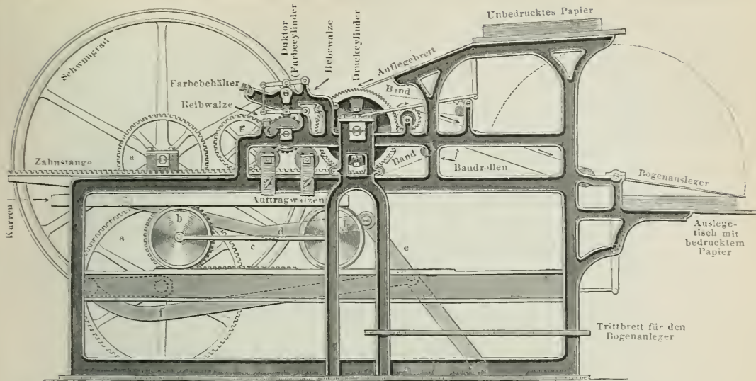
Fig. 1. Ältere Schnellpresse mit Eisenbahnbewegung und einfachem cylindrischen Farbwerk (Ansicht).
