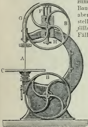
Fig. 17. Bandsäge.
