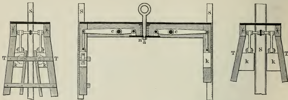
Fig. 15. Fangvorrichtungen mit Klemmbacken.
