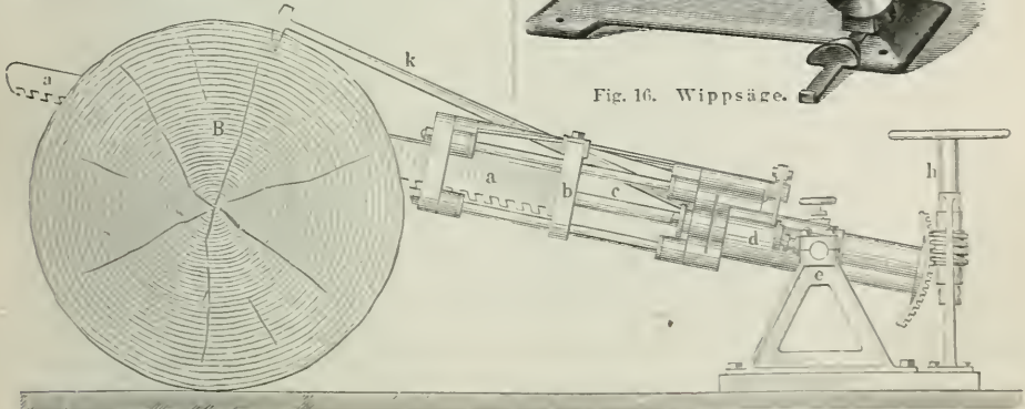
Fig. 15. Dampfquerschneidesäge.
