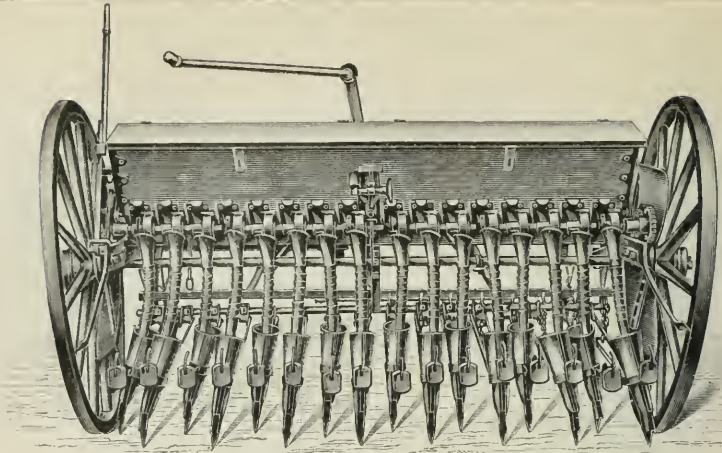
Fig. 4. Bergdrillmaschine 'Hallensis' von Zimmermann.
