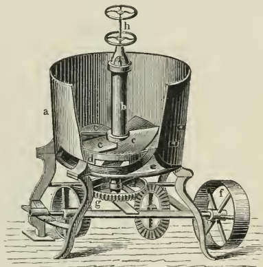
Fig. 10. Amalgamierpfanne.
