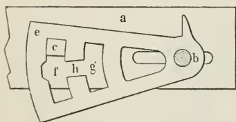
9. Schloßriegel und eine Zuhaltung.
