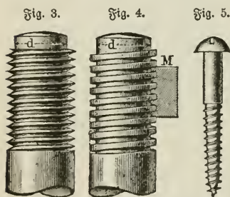
3. Scharfgängige, 4. flachgängige Schraube. 5. Holzschraube.
