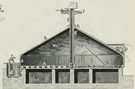
Fig. 10. Rundpfanne mit Rührwerk.
