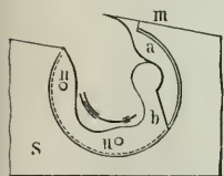
Fig. 9. Auswechselbarer Sägezahn.
