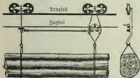
Fig. 3. Längsschnitt der Seilbahn, System Bleichert und Otto.
