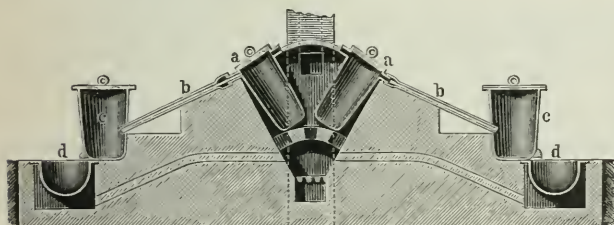
Fig. 2. Sublimation des Schwefels aus gußeisernen Retorten.
