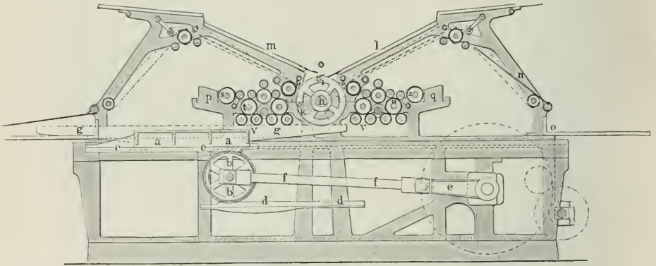
Fig. 6. Durchschnitt der Johannisberger Doppelmaschine.
