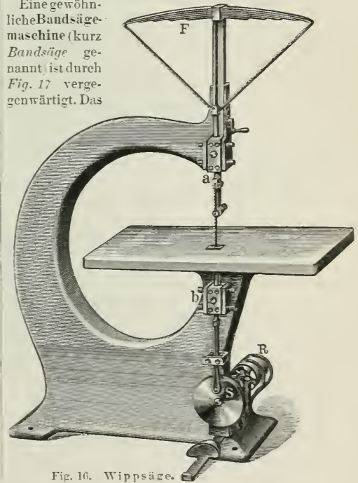
Fig. 16. Wippsäge.
