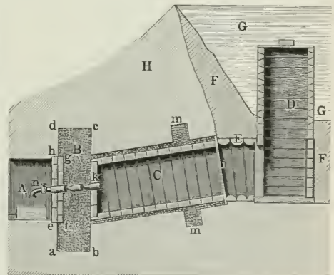
Fig. 5. Wöhrbau.
