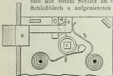
Fig. 2. Schiebende Falle.
