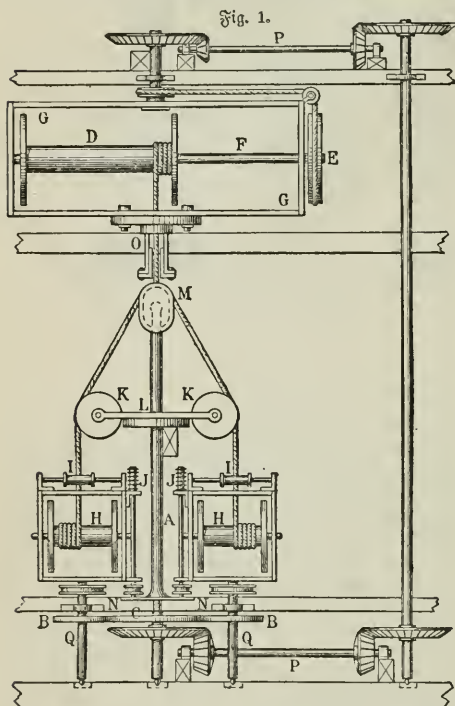
Fig. 1—3. Seilmaschine.
