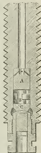
Fig. 3. Nobel's Gasdruckmesser.
