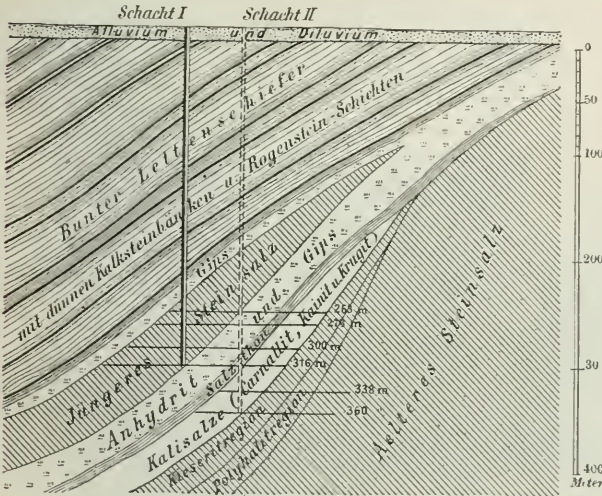
Fig. 1. Gebirgsprofil eines Salzbergwerks bei Staßfurt.
