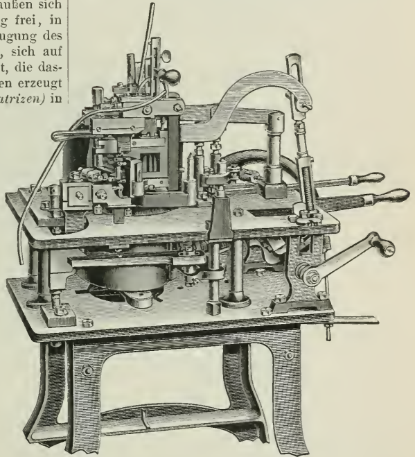
Fig. 1. Einfache Gießmaschine von Küstermann u. Komp. in Berlin.
