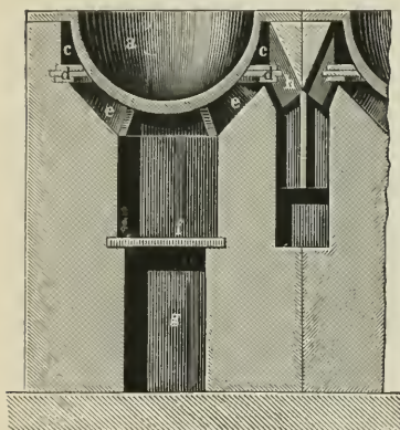
Fig. 7. Pattinsonkessel.
