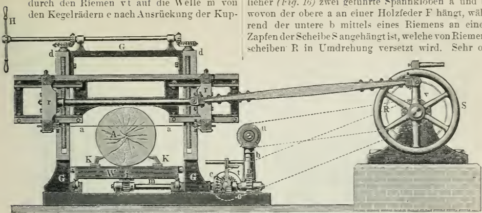
Fig. 14. Horizontalgattersäge.
