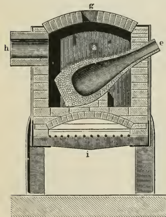
Fig. 8. Vorderansicht im Durchschnitt.
