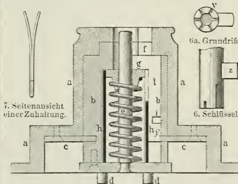
5. Schließcylinder und Zuhaltungen.
