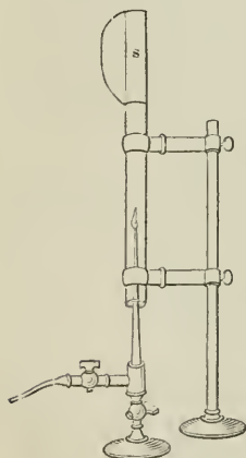
Fig. 10. Singende Flamme.
