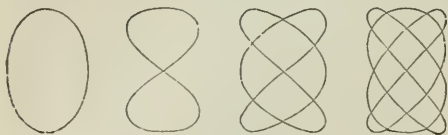
Fig. 18. Lissajous' Schwingungsfiguren.
