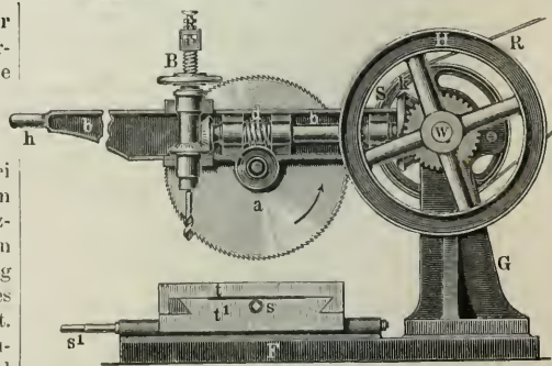
Fig. 22. Kallsäge.
