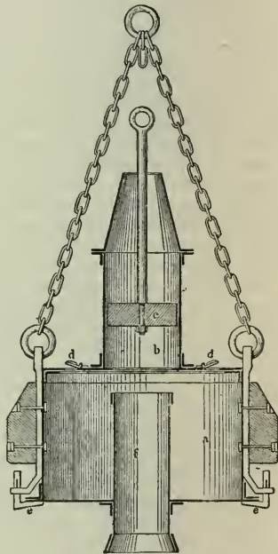
Sandpumpe (Längsschnitt).
