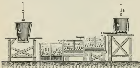
Fig. 12. Apparat für Kochsalzlaugerei.
