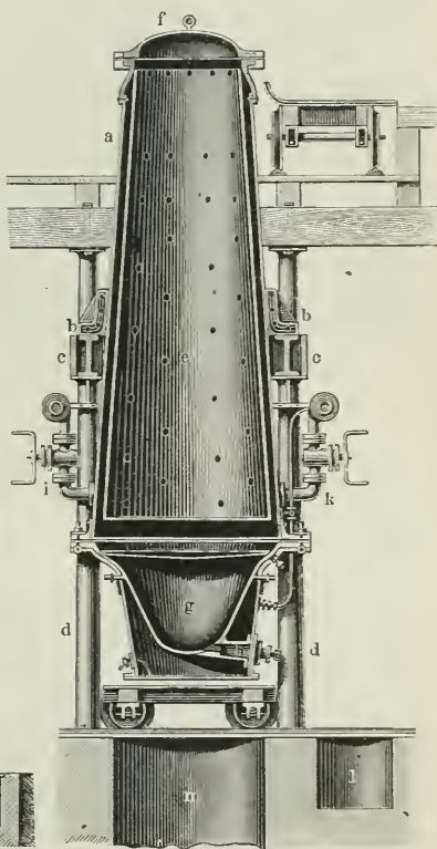
Fig. 3. Grittis Apparat zum Ausschmelzen des Schwefels.
