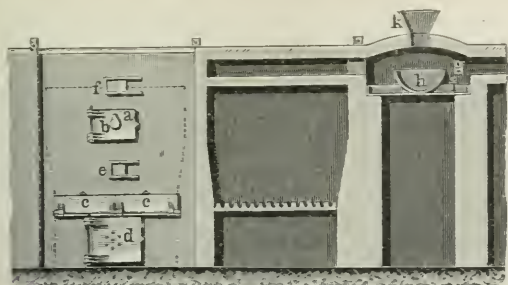
Fig. 1. Ansicht und Längsschnitt.
