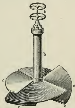
Fig. 11. Läufer der Amalgamierpfanne.
