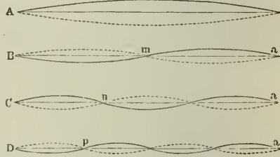
Fig. 11. Schwingungsformen einer Saite.
