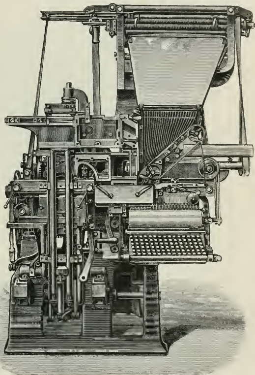
Fig. 1. Linotype.
