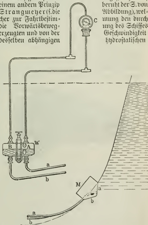
Schiffsgechwindigkeitsmesser von Strangmeyer.
