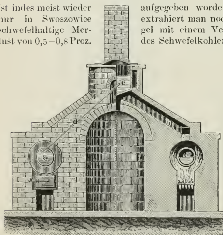
Fig. 5. Querschnitt.
