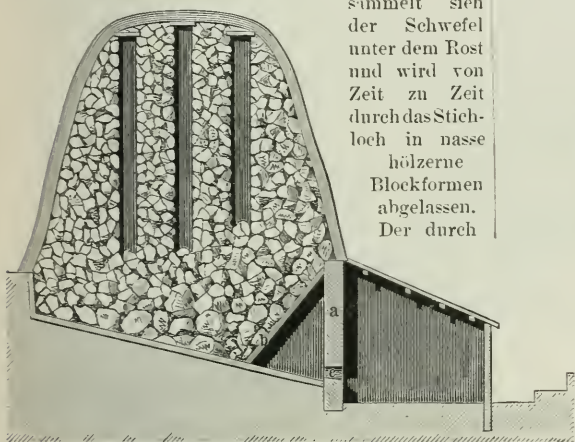
Fig. 1. Meiler zum Ausseigern des Schwefels.
