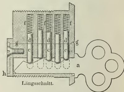
Fig. 12. Yale-Schloß.
