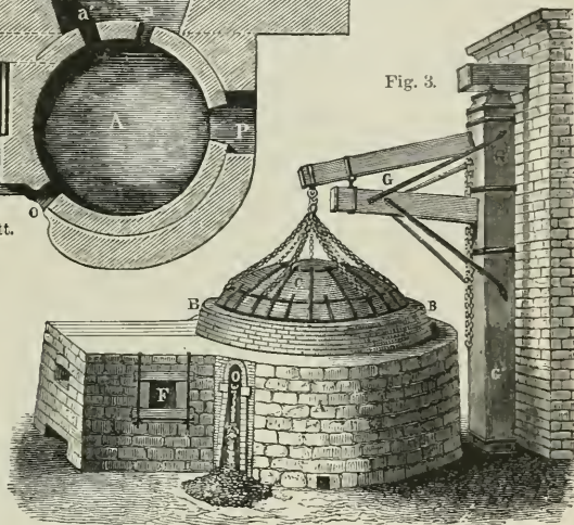
Fig. 1, 2 u. 3. Deutscher Treibherd zum Abtreiben des Bleies.
