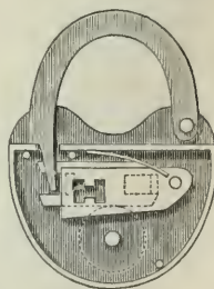
Fig. 11. Chubb-Vorhängeschloß
