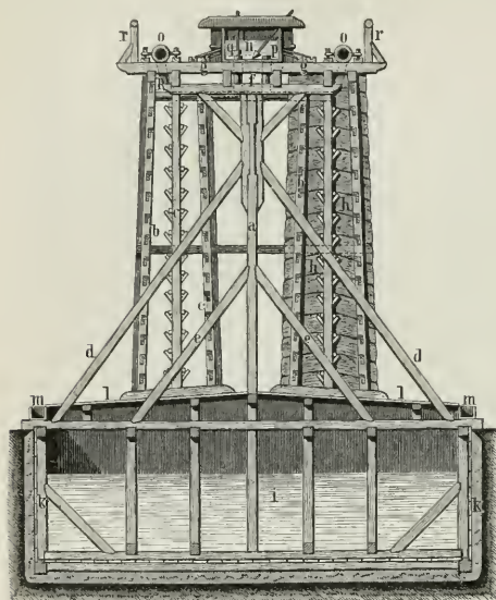
Fig. 6. Dorngradierhaus.
