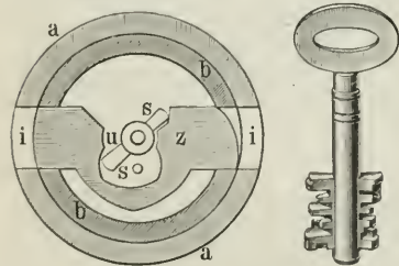
Fig. 20. Zuhaltungsplättchen. Fig. 21. Schlüssel.
