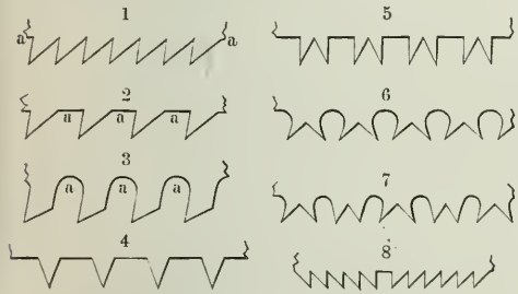
Fig. 1—3. Formen der Sägezähne.
