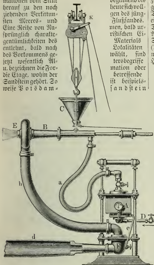
Fig. 1. Sandstrahlapparat mit Dampftrieb.
