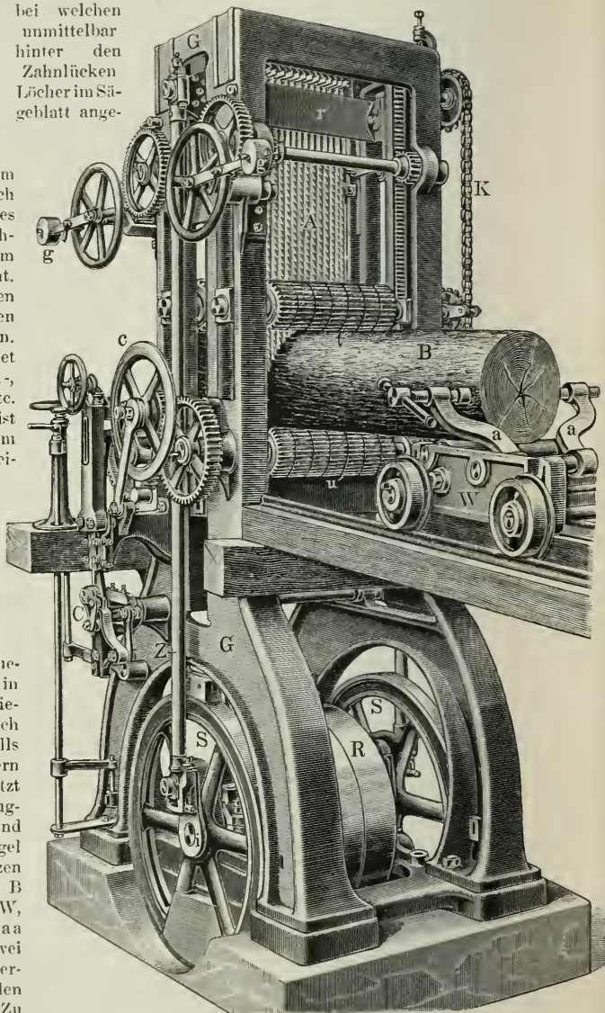
Fig. 13. Vertikalvollgattersäge von Kirchner.
