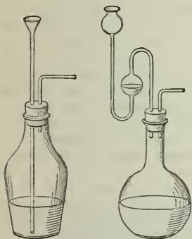
Fig. 1. Sicherheitsröhre.
