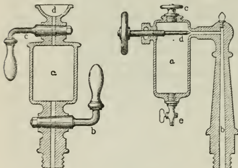
Fig. 2. Schmierhahn. Fig. 3. Kontinuierlich wirkender Schmierapparat.
