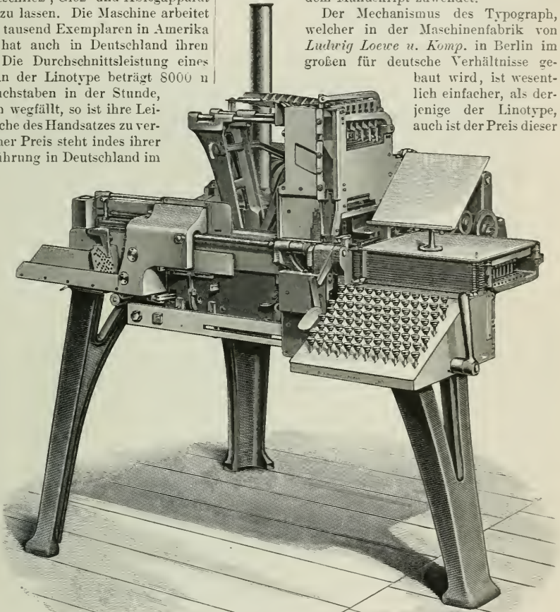
Fig. 4. Monoline.
