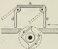
Fig. 10. Schutzvorrichtung an Hobelmaschinen.
