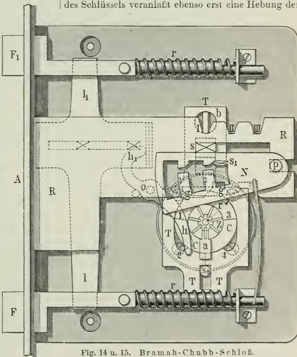
Fig. 14 u. 15. Bramah-Chubb-Schloß.
