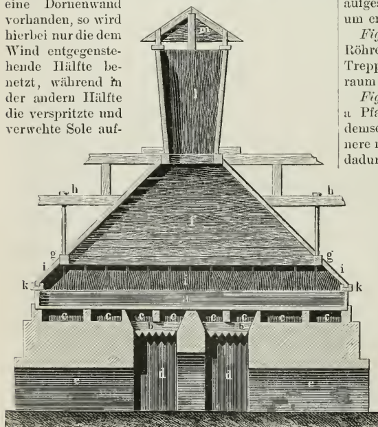
Fig. 7. Siedevorrichtung mit Planrostfenerung.
