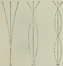
Fig. 13. Schwingungsformen eines am einen Ende eingeklemmten Stabes.
