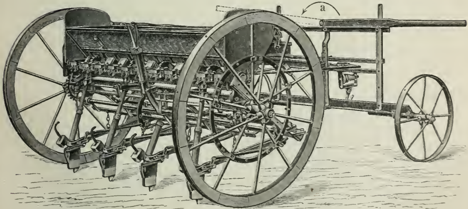
Fig. 3. Drillmaschine Klasse I, vierreihig, mit Klappdibbelapparat für Rübenkerne, von Rud. Sack.
