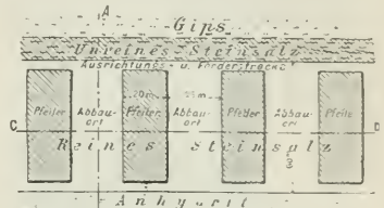
Fig. 2. Grundriß des Örterbaus im jüngeren Steinsalz.
