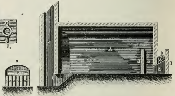
Fig. 13. Dörripfiesel mit Pultfeuerung. a Feuerung.
