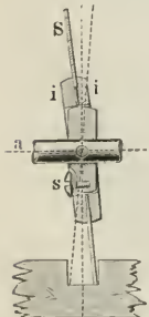
Fig. 21. Taumelsäge.
