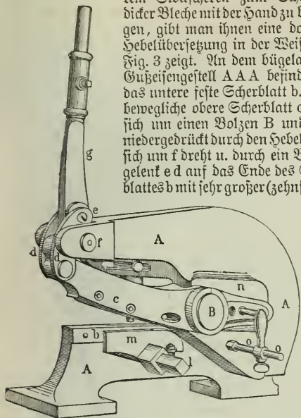
Fig. 3. Bodschere.
