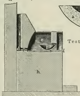
Fig. 6. Muffelofen zum Feinbrennen.
