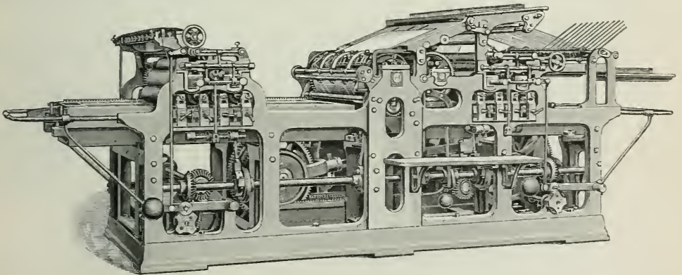
Fig. 2. Zweifarbenschnellpresse von König u. Bauer mit Schlittenbewegung u. Doppelfarbwerken.
