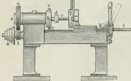
Fig. 11. Schraubenschneidmaschine.
