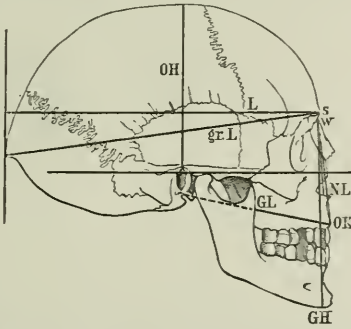
Fig. 2. Langschädel in der Seitenansicht; L gerade Länge; gr. L größte Länge; OK Obergesichtshöhe; GH Gesichtshöhe; GL Profillänge; NL Nasenhöhe; OH Ohrhöhe; s Stirnnaßennast; w Sutura naso-frontalis (Nasennurzel).
