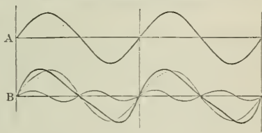
Fig. 24. Schwingungsformen.
