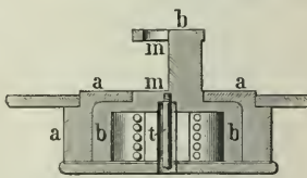
Fig. 19. Zuhaltungsgehäuse.
