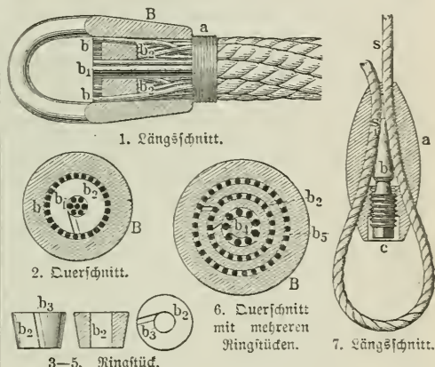
Fig. 1—6. Seilschloß von Keller mit einem Ringstück. Fig. 7. Seilschloß von Strohdach.
