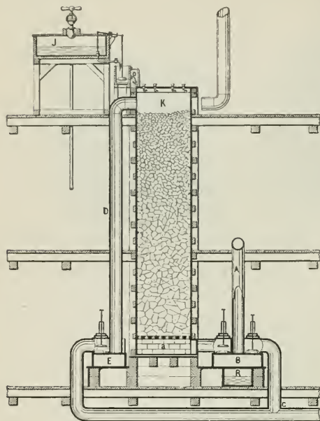
Fig. 5. Gay-Lussacscher Turm.
