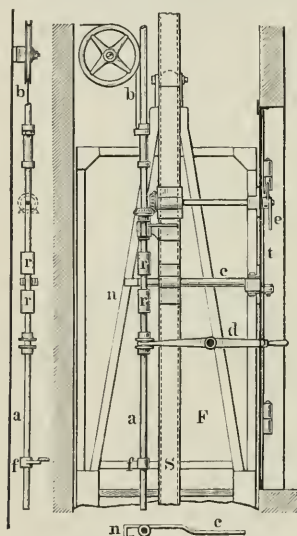
Fig. 16. Thürverschluß an einem Fahrstuhl der Berlin-Anhaltischen Maschinenbaugesellschaft.
