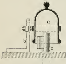
Fig. 9. Schutzglocke an Fräsmaschinen.
