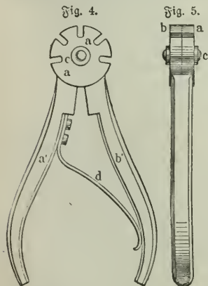
Fig. 4 u. 5. Drahtschere.
