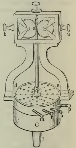
Fig. 3. Sirene.
