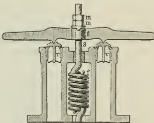
Fig. 2. Sicherheitsventil mit direkter Federbelastung.
