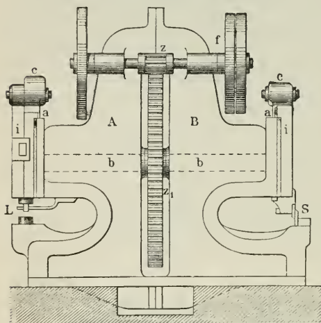
Fig. 7. Loch- und Schermaschine.
