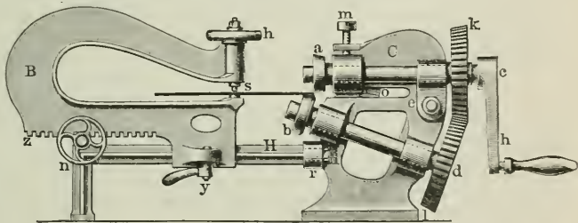
Fig. 6. Kreisschere.
