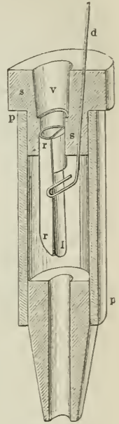
Fig. 16. Zungenpfeife.
