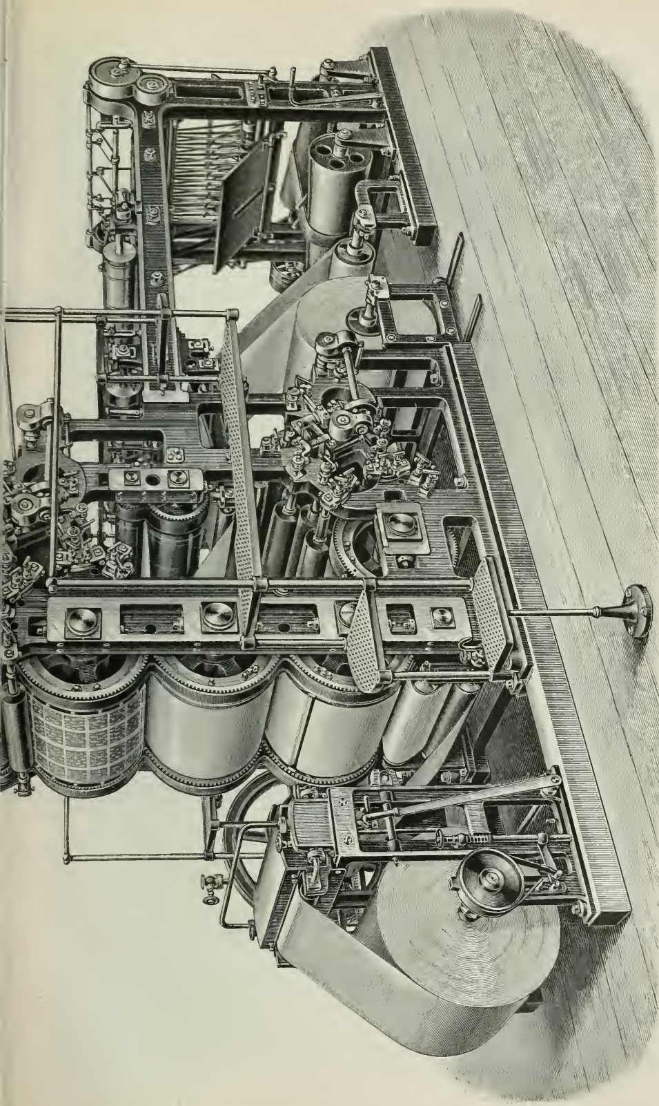
Fig. 5. Rotationsmaschine für Illustrationsdruck. Von der Maschinenfabrik „Augsburg“ für den Druck von „Meyers Konversations-Lexikon“ gebaut. (Beschreibung im Artikel „Schnelldruck“.)
