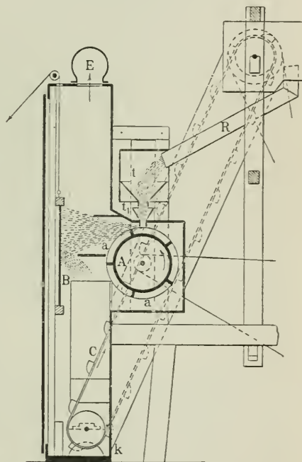
Fig. 2. Sandstrahl-Glaskleifmaschine.
