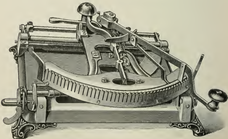
Fig. 4. „Kosmopolit“-Schreibmaschine.
