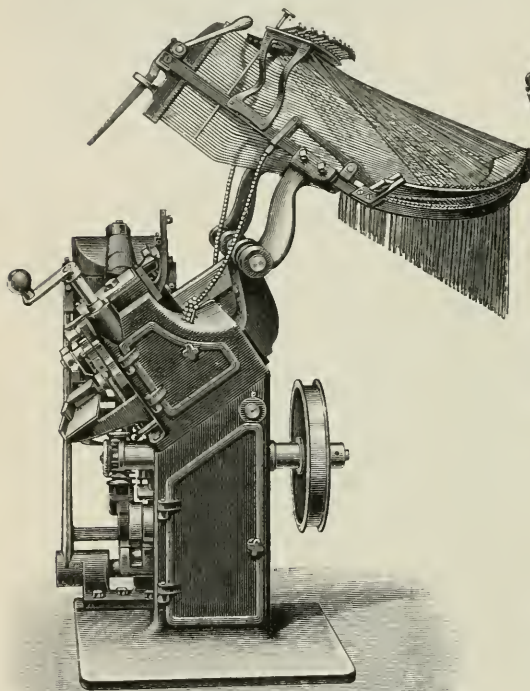
Fig. 2. Typograph mit aufgeschlagenem Rahmen.
