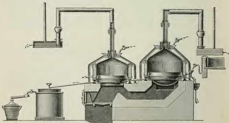
Fig. 6. Verdampfapparat von Faure u. Kehler.
