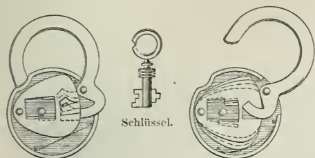
Geschlossen. Geöffnet. Fig. 13. Steinkes Vorhängeschloß.
