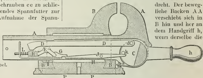
Fig. 14. Halls Parallelschraubstock (Schnitt).
