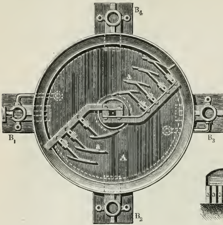
Fig. 12. Mechanische Dampfsalzdarre.
