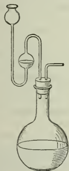
Fig. 1. Sicherheitsröhre.
