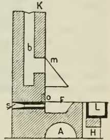
Fig. 1. Schmiedeherd.
