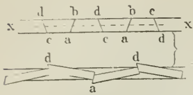
Fig. 11. Schärfen der Sägen.
