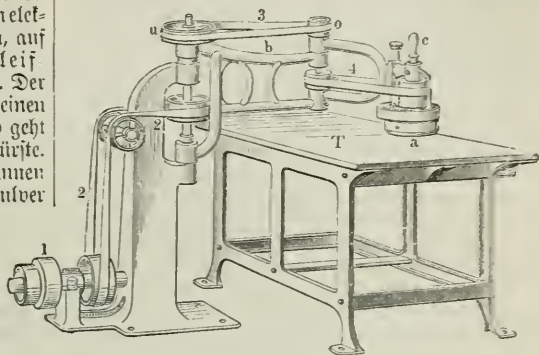
Fig. 2. Sandschleifmaschine.
