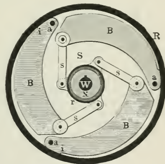
Fig. 14. Schleuderbremse.
