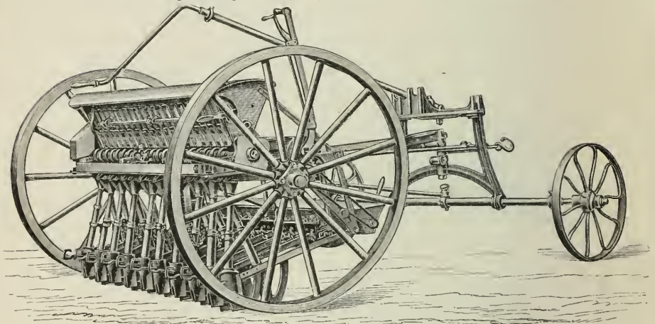
Fig. 5. Nutenwalzen-Drillmaschine 'Berolina' mit Kleesäeapparat, von Eckert.
