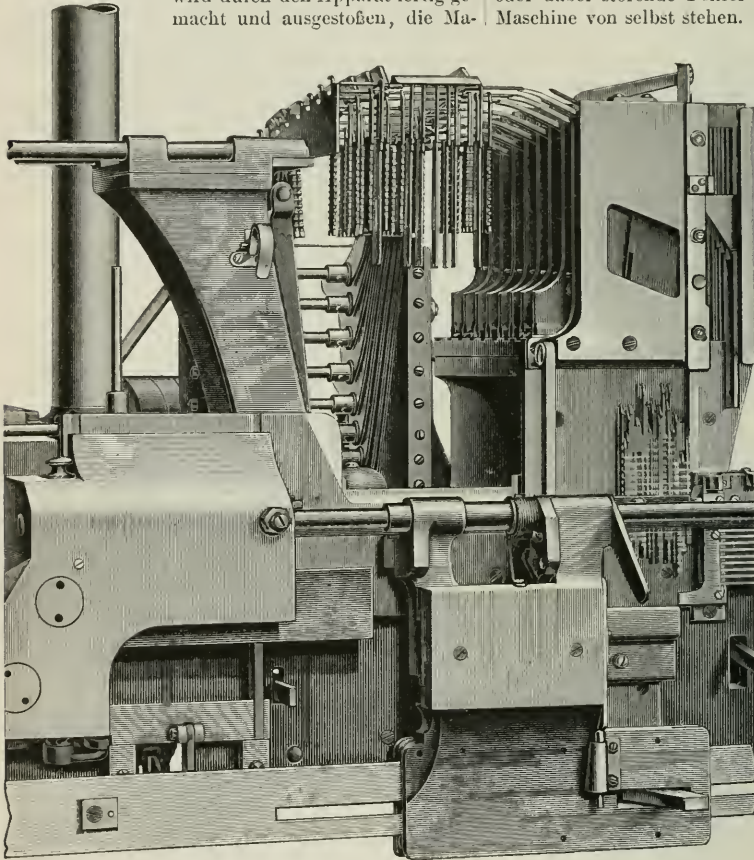
Fig. 5. Matrizen-trägermagazin der Monoline.
