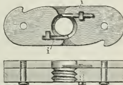
Fig. 8. Schneidzeug für hölzerne Schrauben.
