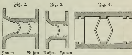
Fig. 2. Schutz- oder Sperrschleuse. Fig. 3. Dockschleuse. Fig. 4. Verbindung von Schutz- und Dockschleuse.
