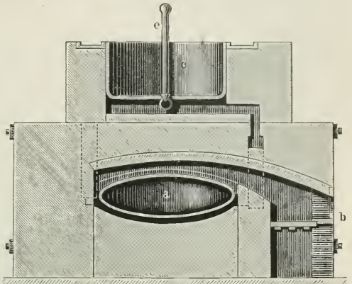
Fig. 7. Längsschnitt.
