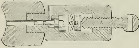
Fig. 1. Rodmans Gasdruckmesser.
