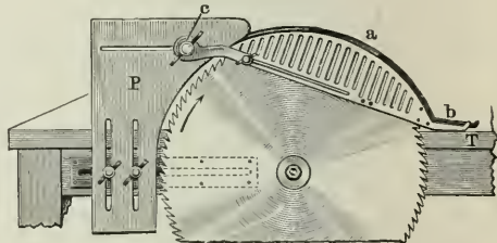
Fig. 11. Schutzhaube an Kreissägen von Kirchner.
