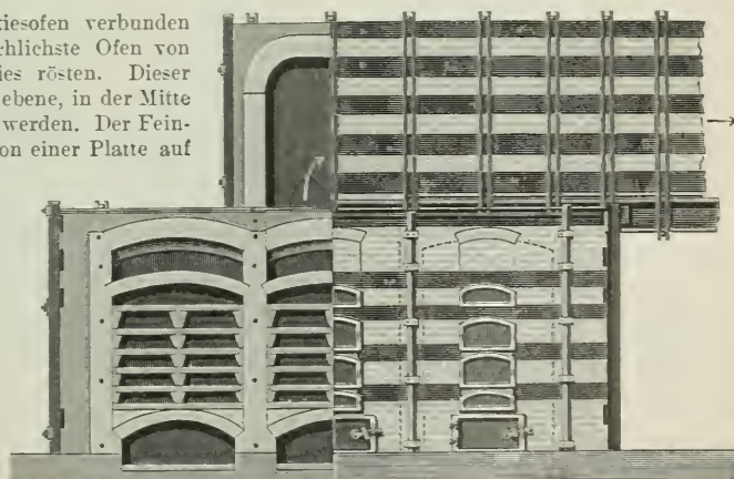
Fig. 3 u. 4. Malétraofen.
