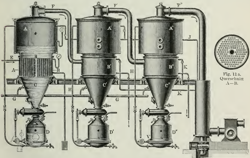
Fig. 11. Pickseher Verdampfapparat, der erste Körper im Durchschnitt.
