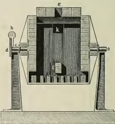
Fig. 8 u. 9. Zinkdestillierofen.
