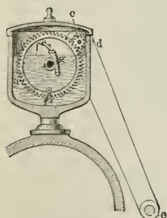
Fig. 4. Mechanische Schmier- vorrichtung.
