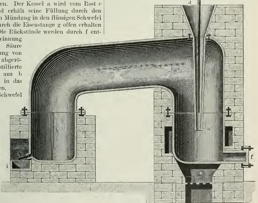
Fig. 8. Deutscher Apparat zur Raffination des Schwefels.
