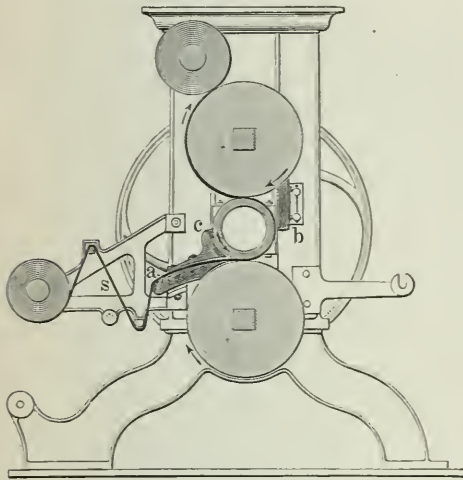
Fig. 12. Fingerschutz an Kalandern.
