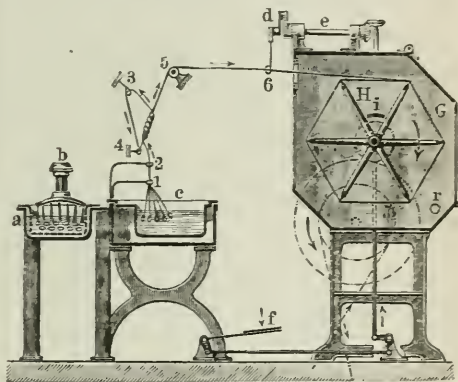
Seidenhaſpel
