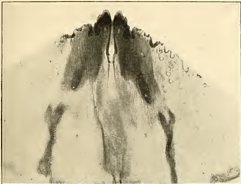
FIG. 1.—ASPIDIOTUS (DIASPIDIOTUS) TRANSCASPIENSIS.
