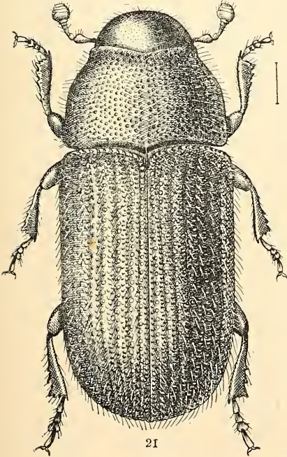
Fig. 17.— D. obsesus . Fig. 18.— D. rufipennis . Fig. 20.— D. punctatus . Fig. 21.— D. micans . (Original.)
