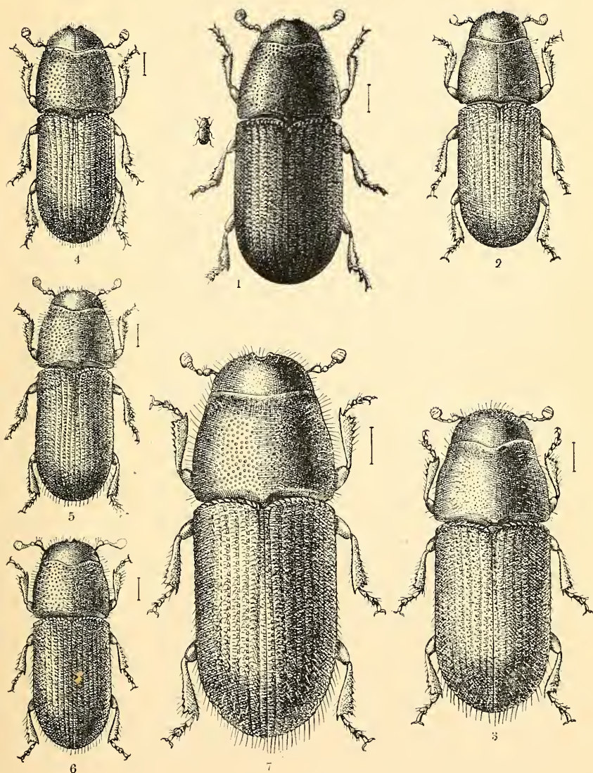
Fig. 1.— D. brevicornis . Fig. 2.— D. barberi . Fig. 3.— D. convexifrons . Fig. 4.— D. frontalis . Fig. 5.— D. arizonicus . Fig. 6.— D. mexicanus . Fig. 7.— D. parallellocollis . (Original.)
